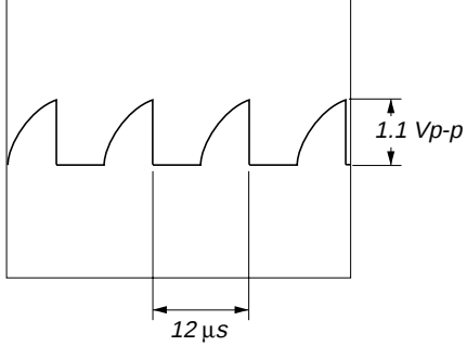
❺ IC700 ⑦③ (XOA)
