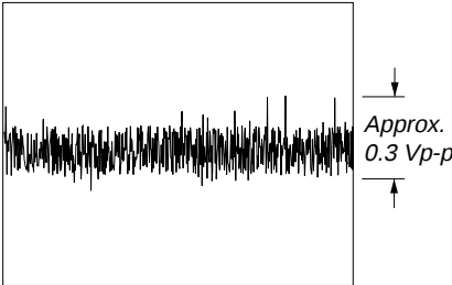
❷ IC302 ③④ (FE) (MD PLAY Mode)
